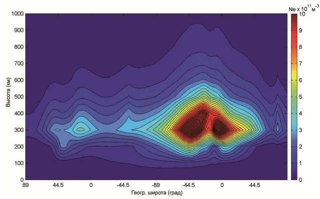
Рис. 3. Модельное распределение электронной концентрации в ионосфере для элемента реконструкции 50 \times 100 км
