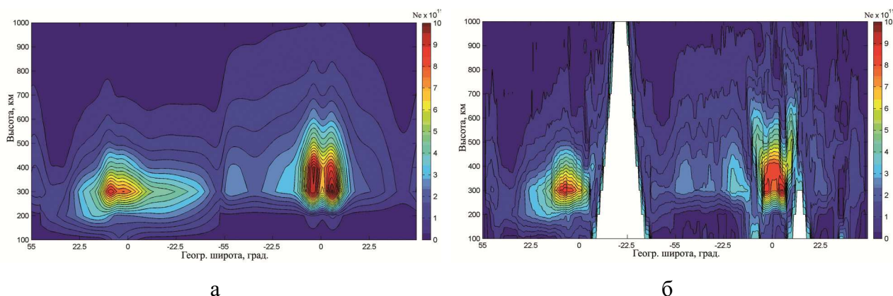
Рис. 1. Распределение электронной концентрации в ионосфере в плоскости орбиты ГНСС в координатах широта – высота над уровнем моря, цветом кодированы значения электронной концентрации ( 10^{11} эл.м -3 ); а – модельное распределение, б – реконструкция, полученная при использовании в качестве источников сигнала 5 КА GPS и 6 КА ГЛОНАСС
