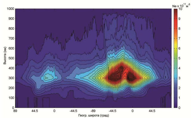
Рис. 6. Реконструкция модельного распределения (рис. 3) электронной концентрации с использованием четырех кластеров из 4 КА за период 20 минут с использованием начального приближения
