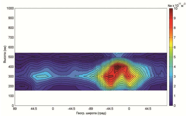
Рис. 4. Реконструкция модельного распределения электронной концентрации в ионосфере (рис. 3) с использованием кластера из 4 КА за 1 виток без использования начального приближения
