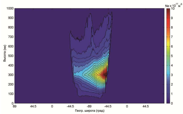
Рис. 5. Реконструкция модельного распределения электронной концентрации (рис. 3) с использованием одного кластера из 4 КА за период 15 минут с использованием начального приближения
