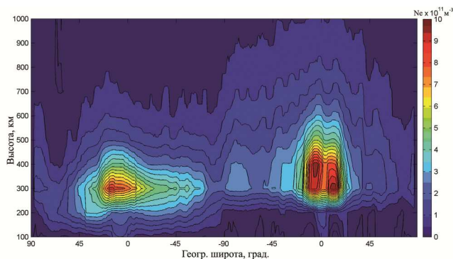
Рис. 2. Распределение электронной концентрации в ионосфере в плоскости полярной орбиты в координатах широта-высота. Реконструкция по данным от модельной группировки из 36 КА. Время экспозиции 15 минут.
