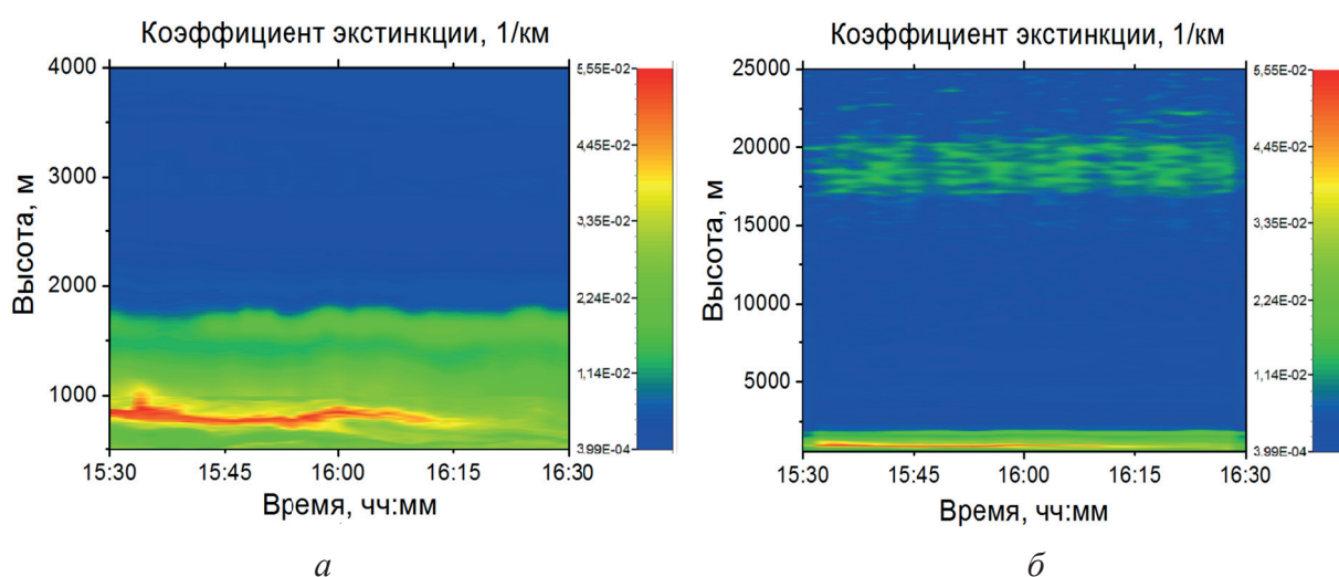
Рис. 2. Временная зависимость изменчивости вертикального профиля объемного коэффициента ослабления в слое атмосферы а) 0–4 км и б) 0–25 км по результатам обработки сигнала обратного рассеяния, зарегистрированного в лидарном зондировании 25.03.2013 в центре Санкт-Петербурга. Шкала справа показывает значение коэффициента ослабления в \text{км}^{-1}
