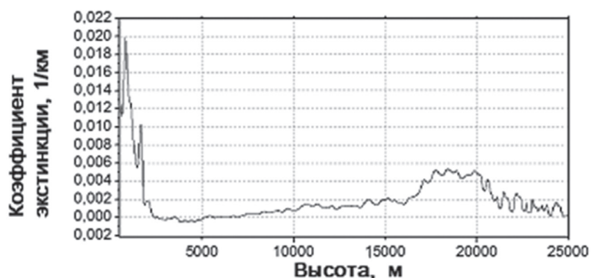
Рис. 1. Зависимость объемного коэффициента ослабления в безоблачной атмосфере, усредненного за 1 час, по результатам обработки сигнала обратного рассеяния, зарегистрированного в лидарном зондировании 25.03.2013 в центре Санкт-Петербурга
