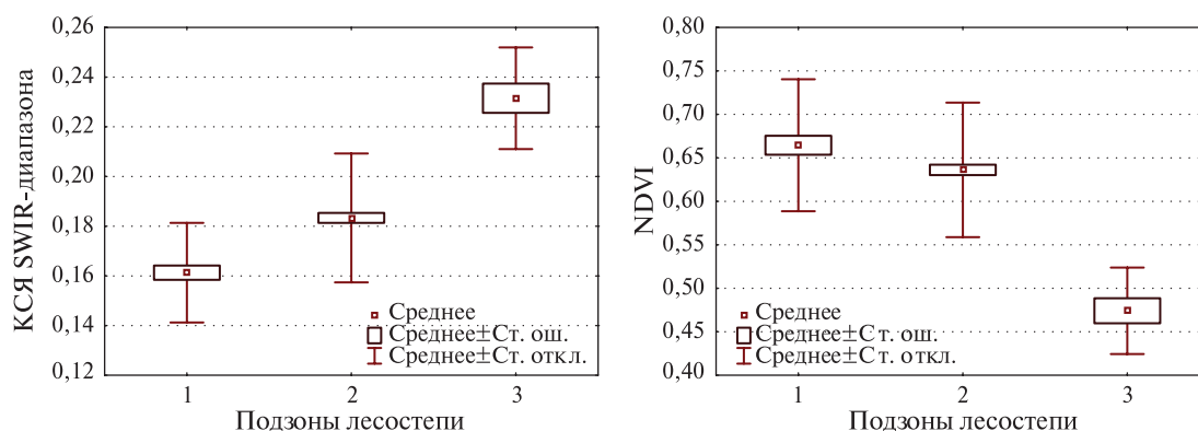
Рис. 3. Значения спектрально-отражательных характеристик залежных земель (по Landsat-8 OLI) с листовыми породами для подзон северной (1), типичной (2) и южной (3) лесостепи (2018)
